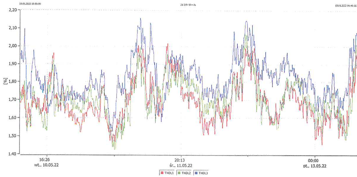
Wykres 3. THDU
