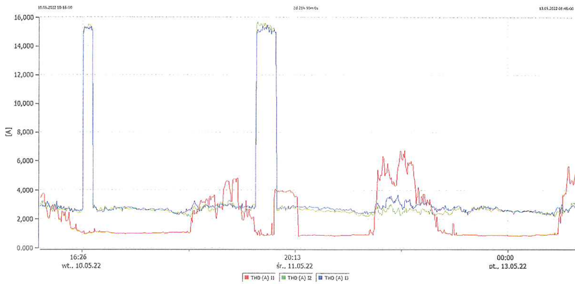
Wykres 4. THDI
